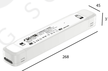
24V 150W FULHAM
